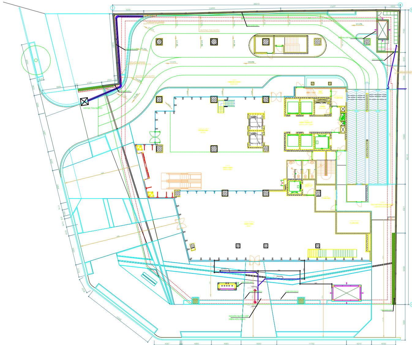
MẶT BẰNG BỐ TRÍ THOÁT NƯỚC KHU LANDSCAPE LAYOUT PLAN DRAINAGE ZONE LANDSCAPE
